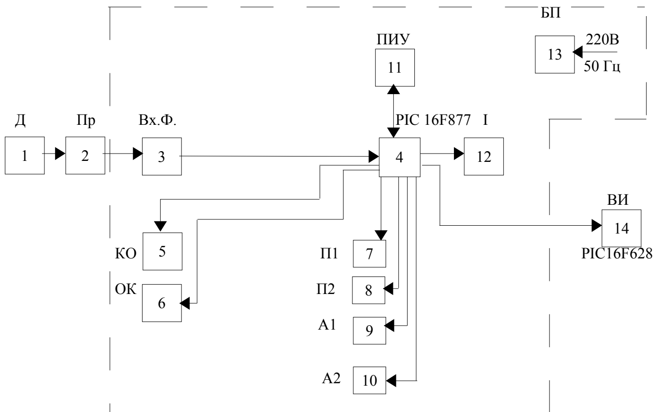
Рис. 1 Структурная схема тахометра ИП-114/60.
