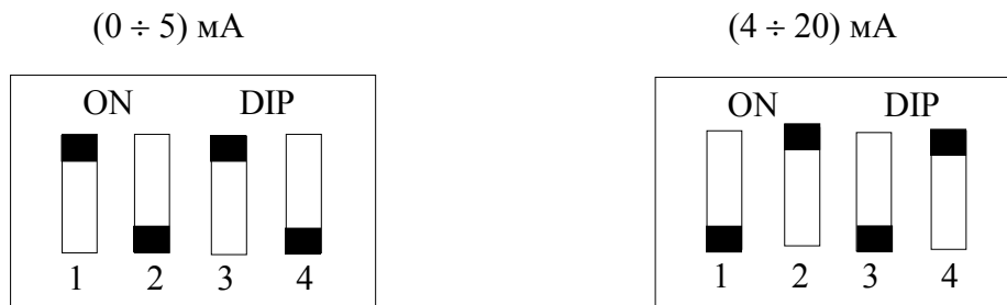
Положение DIP-переключателей
